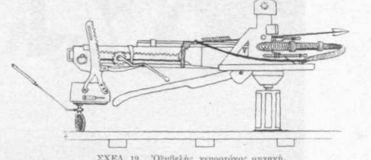
ΣΧΕΔ. 19. Ὁμοειδῆς νευροτόνος μηχανή.
