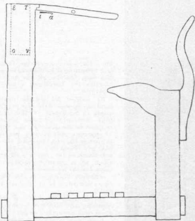
ΣΧ. 1.— Τὸ Ἀθηναϊκὸν θρανίον Ἐ. Μιχαλοπούλου. Κατακόρυφος τομή, δεκνύουσα τὴν θέσιν τοῦ γραφείου καὶ τὸ σχῆμα τοῦ ὅλου θρανίου κατὰ τὴν περίπτωσιν τῆς γραφῆς. Διάστημα ἁρνητικῶν = 0,05. Κλίσις 1/10°.
