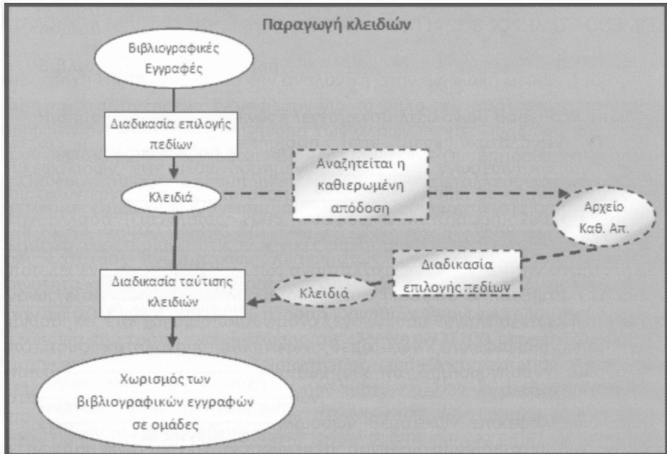
Σχήμα 2: Διαδικασίες δημιουργίας κλειδιών ταύτισης (χωρίς ή με χρήση Αρχείου Καθιερωμένων Αποδόσεων)
