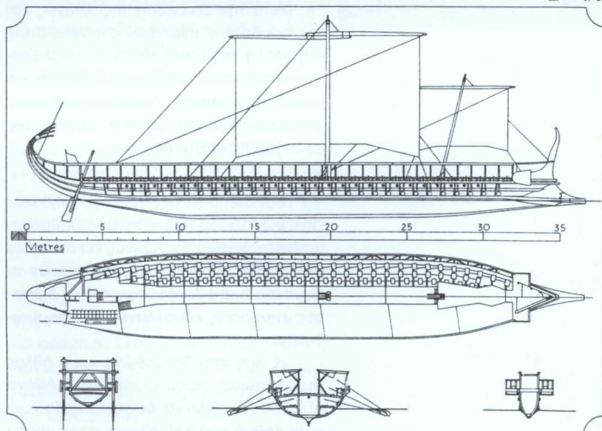
Τριήρης ( http://pages.uoregon.edu/klio/maps/gr/trireme_plan.jpg )
