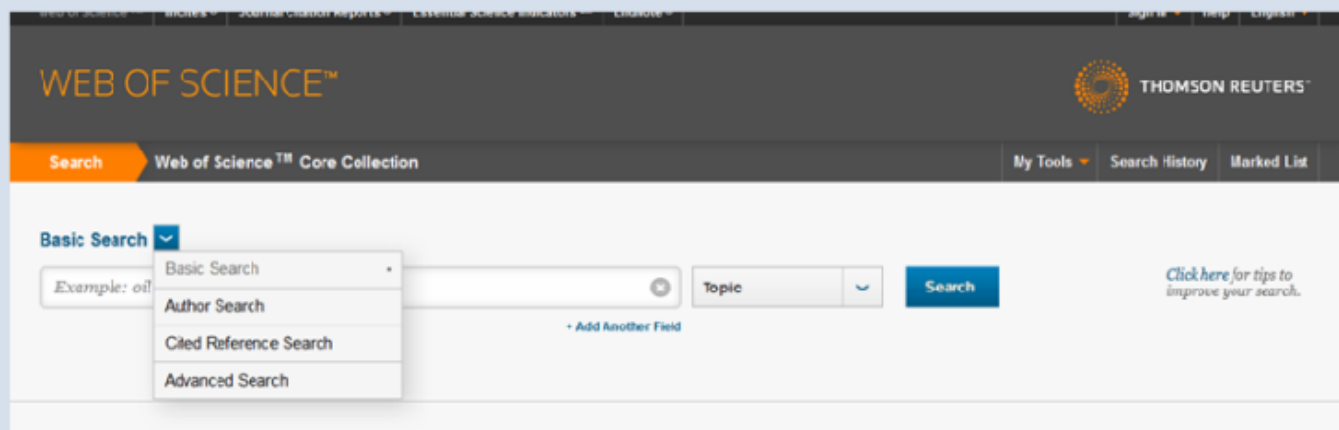
Εικόνα 1: Μηχανισμοί αναζήτησης
