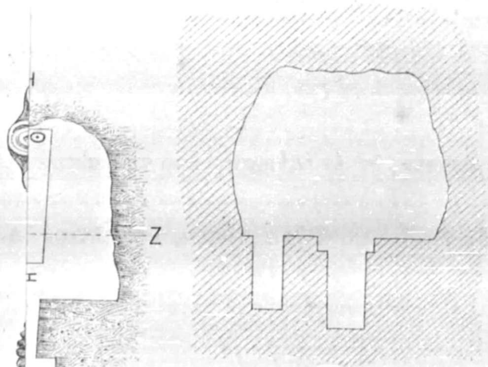
Κατατομὴ κατὰ τὴν Ε-Ζ
