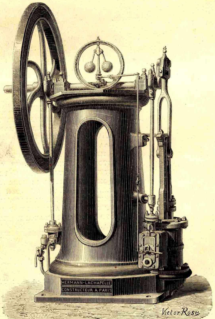
ΝΕΑ ΑΤΜΟΚΙΝΗΤΟΣ ΟΡΘΙΑ ΚΑΙ ΠΕΠΗΓΥΙΑ ΜΗΧΑΝΗ ΤΩΝ Κ. Κ. HERMANN LACHAPELLE EN ΠΑΡΙΣΙΟΙΣ. Faubourg Poissonnière 144.
