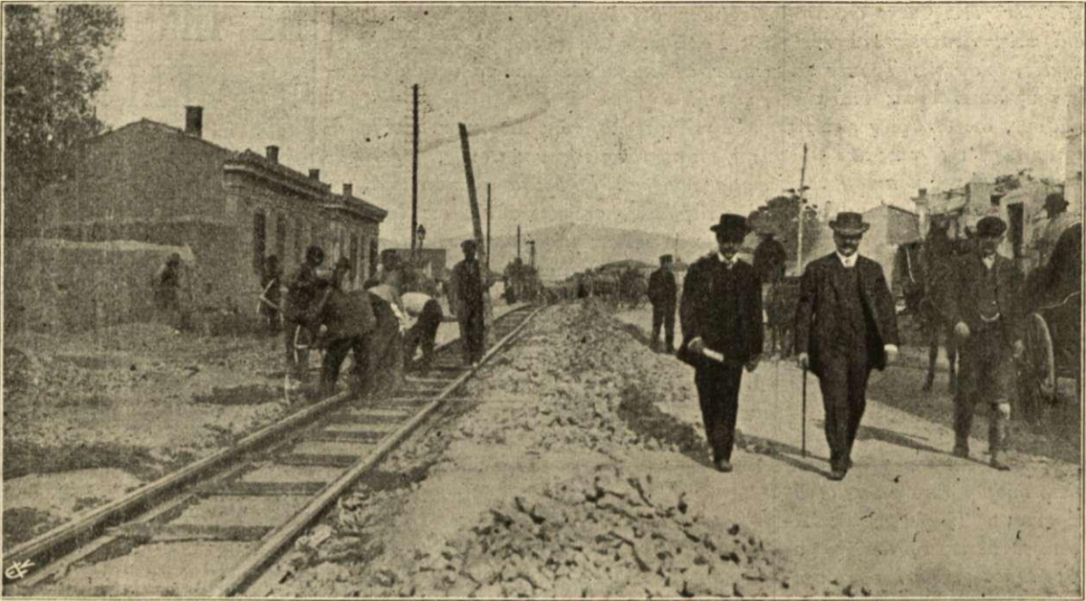
Έργαται στρώνοντες τας σιδηράς ράβδους των ήλεκτρικών τραμ επί της όδου Θ. Δεληγιάννη (πρώην Πελοποννήσου) προς τους σιδηρ. σταθμ. Είς τὸ μέσον της όδου ο κ. Δούμας, διευθυντ. της κατασκευής των τραμ και δεξιὰ του ο κ. Σκέμπερ μηχαν. της Έταιρίας
