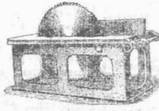
Κυλινδρικός πρίων
