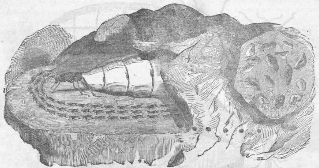
Ἀρχιτεκτονικὴ λευκομυρμηκῶν.
