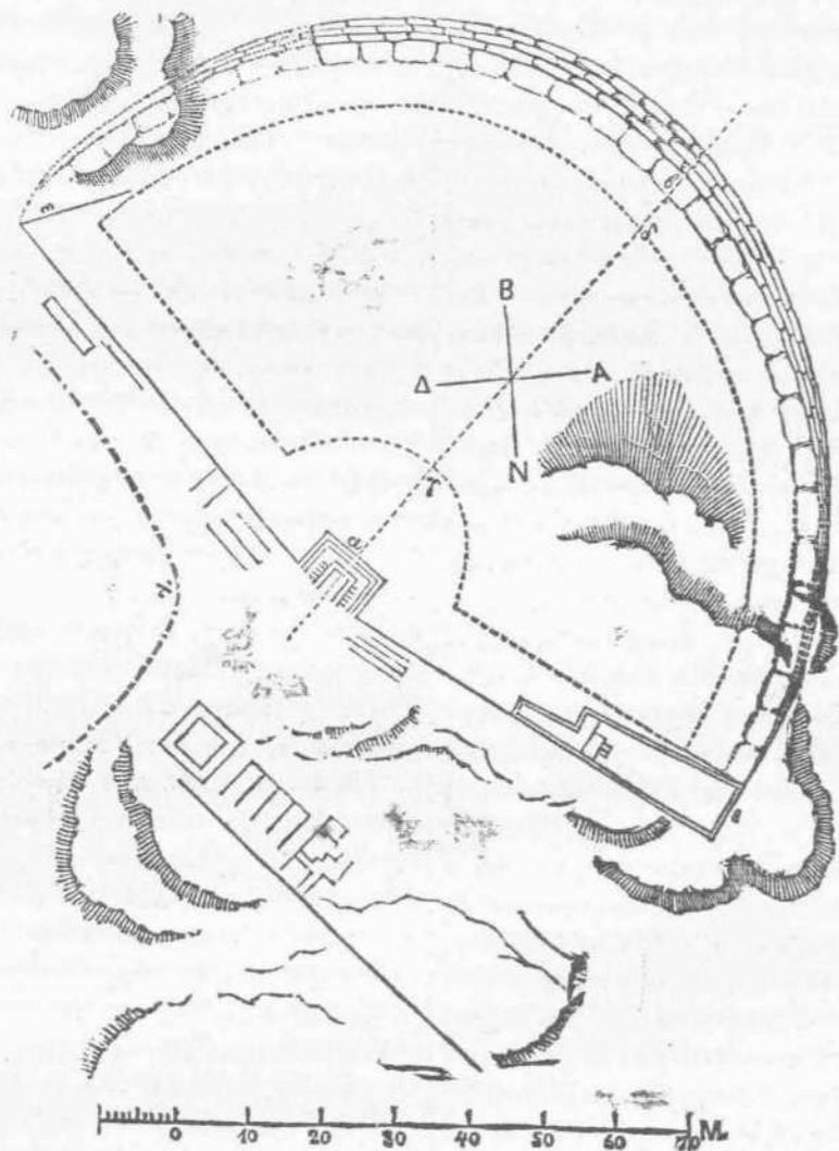
Ἀutoσχεδίασμα τῆς Πρυκὸς.
