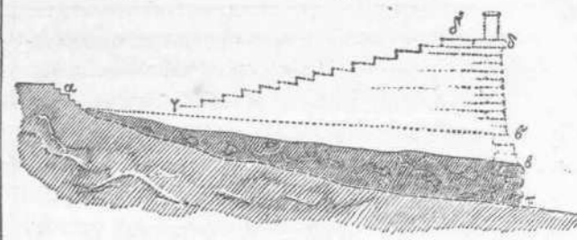
Σχῆμα 2, τομὴ τῆς Πρυκὸς κατὰ τὸ ἀβ. (Σχ. 1) διὰ τῆς αὐτῆς κλίμακος.
