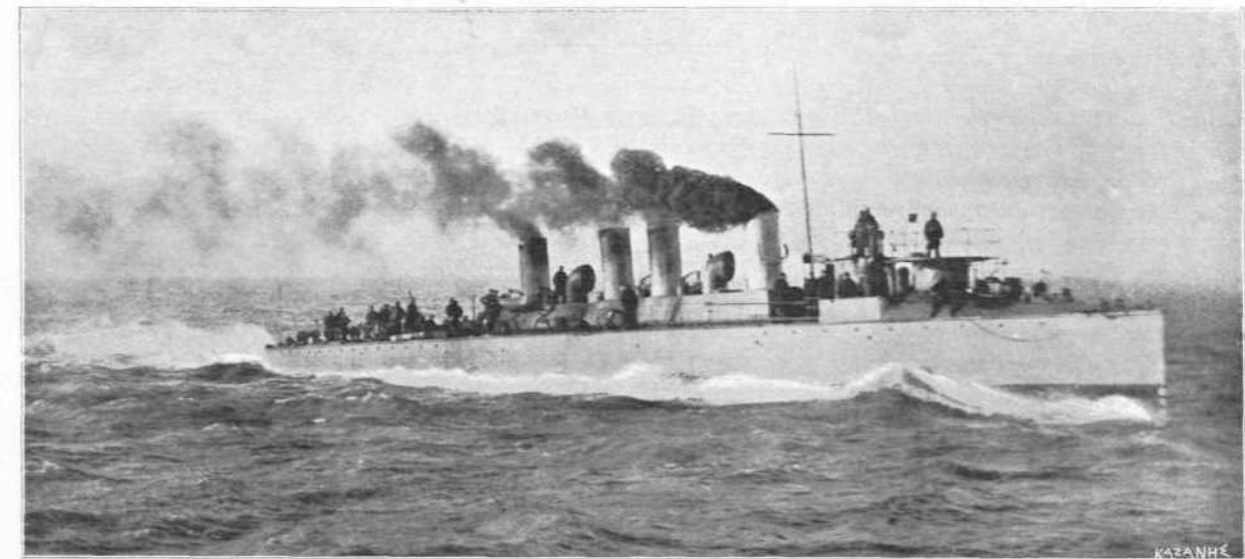
ΤΟ ΙΑΠΩΝΙΚΟΝ ΑΝΤΙΤΟΡΠΙΛΙΚΟΝ "ΣΑΖΑΝΑΜΙ", ΚΑΤΑ ΤΟΝ ΤΥΠΟΝ ΤΟΥ ΟΠΟΙΟΥ ΘΑ ΝΑΥΠΗΓΗΘΟΥΝ ΤΑ ΝΕΑ ΣΚΑΦΗ ΜΑΣ Τὸ «Σαζανάμι» συνέλαβεν αἰχμάλωτον τὸν Ρώσσον ναύαρχον Ροζεδσβένοβι κατά τὴν τελευταίαν ναυμαχίαν.
