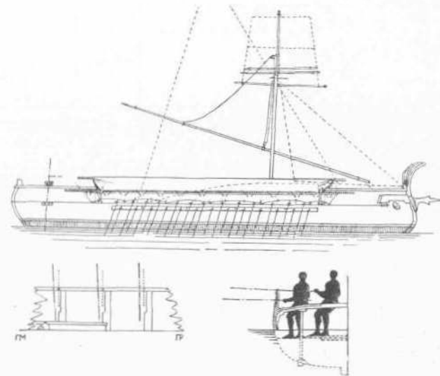
ΣΧΕΔ. 4. Τύπος πλοίου Έρυθραίον.
