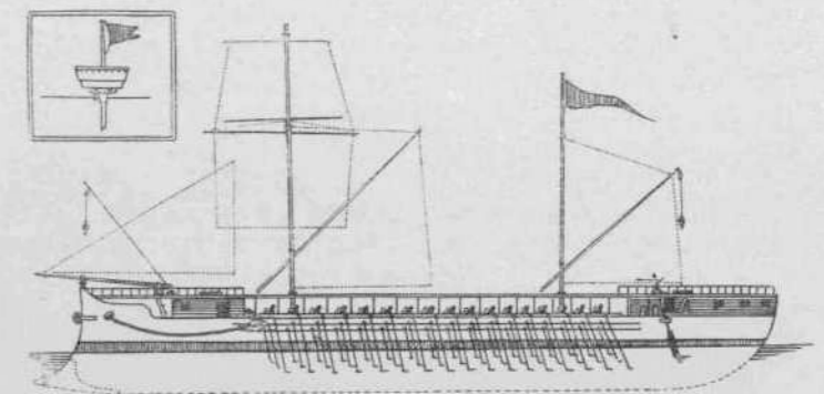
ΣΧΕΔ. 2. Τριήρης της έποχής τού Πελοποννησιακού πολέμου.
