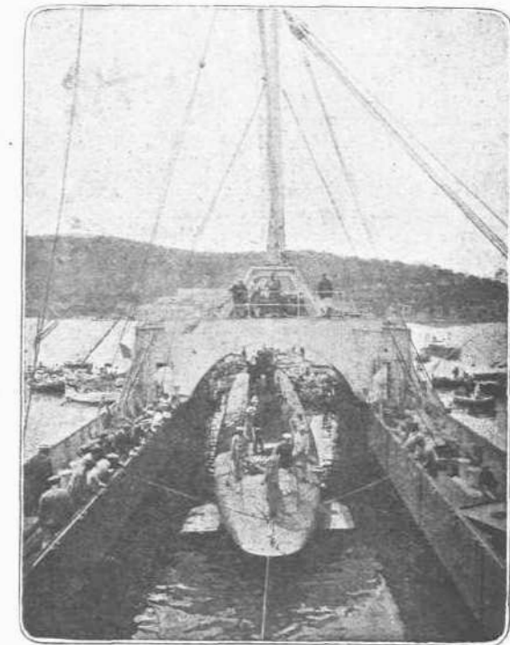
ΚΑΙ Η ΑΝΤΙΘΕΣΙΣ. — Ἴδου και ἡ ἀντίθεσις τώρα. Πρὶν ἡ κατασκευασθῶν τὰ μεγάλα Γερμανικὰ ὑπερωκεάνεια ὑποβρύχια ἡ μεταφορὰ των εἰς μεγάλας ἀποστάσεις εἰναι δι' αἰμοκλιῶν ειδικῶν, όπως αὐτὸ που παρουσιάζει ἡ παρατιθέμενη εἰκὼν. Τὸ κύτος του πλοίου αὐτοῦ είναι κενόν έντελῶς, διά καταλήλει δὲ μηχανισμοῦ βυθίζεται έντός του ὕδατος μέχρις ὄρισμένου σημείου, εἰς τὸ όποιον ὑπάχει ὀπή, διά τῆς όποιᾶς εἰσέρχεται τὸ ὑπερβύχιον.
