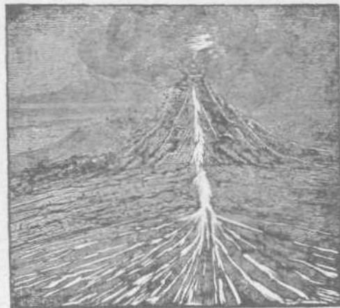
Τομὴ ἠφαιστείου.
