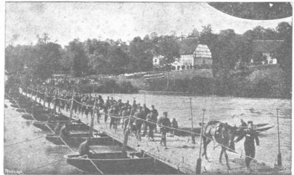
ΤΟΠΟΘΕΤΗΣΙΣ ΚΑΙ ΔΙΕΛΕΥΣΙΣ ΓΕΦΥΡΑΣ ΕΠΙ ΠΟΤΑΜΟΥ
