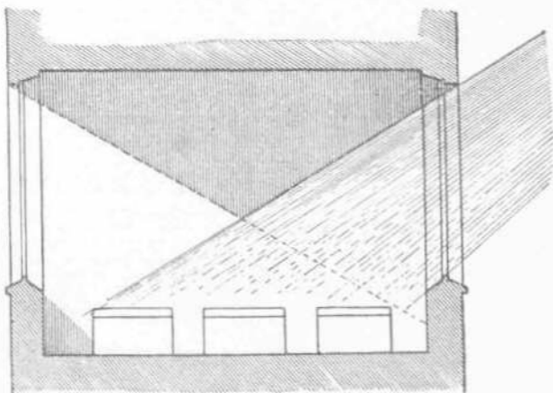
ΑΜΦΟΤΕΡΩΘΕΝ ΦΩΤΙΣΜΟΣ
