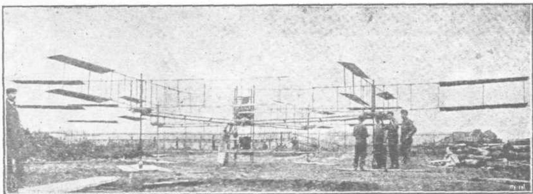
ΤΟ ΒΛΙΚΟΠΤΕΡΟΝ BRÉGUET ΤΟ ΠΡΩΤΟΝ ΑΝΥΨΘΕΝ ΜΕΘ' ΕΝΟΣ ΕΠΙΒΑΤΟΥ
