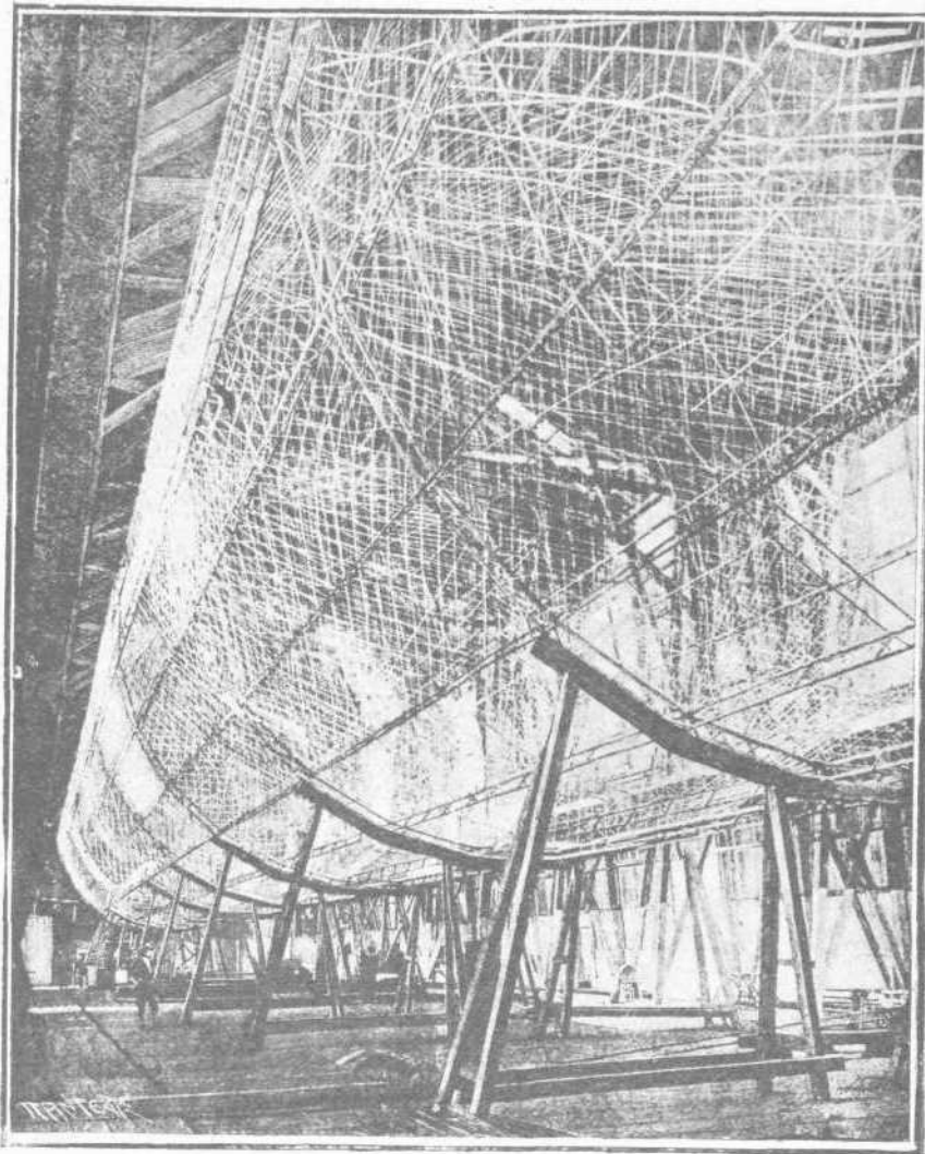
ΠΩΣ ΚΑΤΑΣΚΕΥΑΖΟΝΤΑΙ ΤΑ ΑΕΡΟΣΤΑΤΑ Το εσωτερικόν του πηδαλιουχομένου Ζέππελιν.
