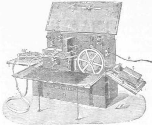
Συσκευή ἀουρμάτου Τηλεγράφου
