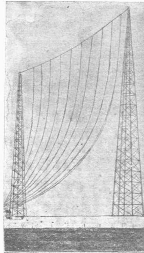
Σταθμὸς ἐν Καζαμπλάκα ἰδρυθεὶς τῷ 1908 και ἐπικοινωνῶν μετὰ τοῦ Πύργου τοῦ Ἄϊφελ.
