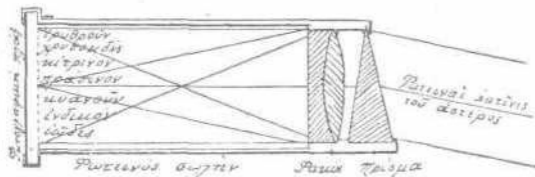
Σχῆμα ἀστρικοῦ φασματοσκοπίου.
