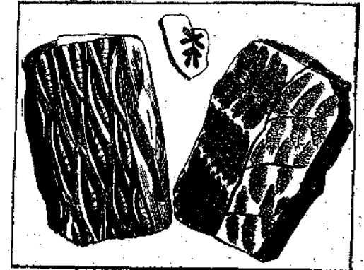
Αποτυπώματα φυτών επί λιθωνθράκων.
