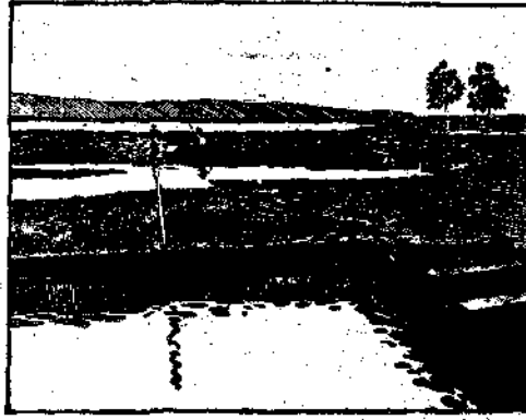
Εἰκὼν 8. Ἀνθρακωρυχία. Τὰ ἀνθρακωρυχία σχηματίζονται ὑπὸ τῆς ἀποσυνθέσεως τῶν φυτικῶν λειψάνων. Ὅταν ὁ ἀνθραξ καίεται, ἀποδίδει ὑπὸ σχῆμα θερμότητος τὴν ἡλιακὴν ἐνέργειαν, ἢν ἀπερρόφησαν τὰ φυτὰ ταῦτα, ὁπόταν συνήκωσαν αὐτὴν μετὰ τοῦ ἀνθρακος, ὃν ἔφερον.
