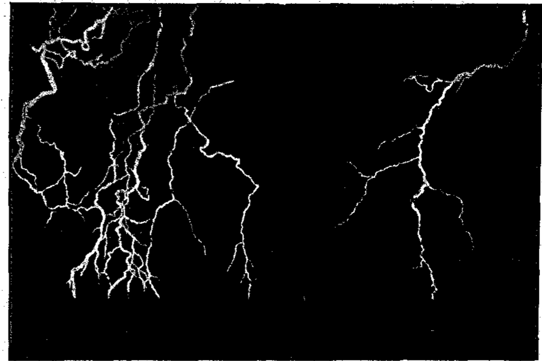
Συνεχεῖς ἐκκενώσεις μεταξὺ νεφῶν καὶ γῆς.
