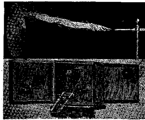
Εἰκ. 7. Ἡλεκτρικὴ ἐκκένωσις μεταξὺ αἰχμῆς καὶ δίσκου. Κάτωθι κινηματογραφικὴ μηχανή.
