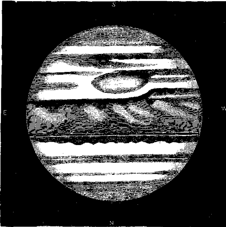
Ὁ πλανήτης Ζεύς.
