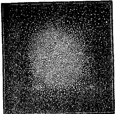
Σπορὸς ἀστέρων : πλησίον τοῦ Ἀστερισμοῦ ω Κενταύρου.
