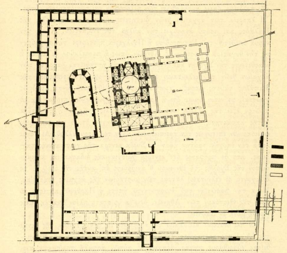
ΔΙΑΓΡΑΜΜΑ ΤΗΣ ΜΟΝΗΣ ΔΑΦΝΙΟΥ
