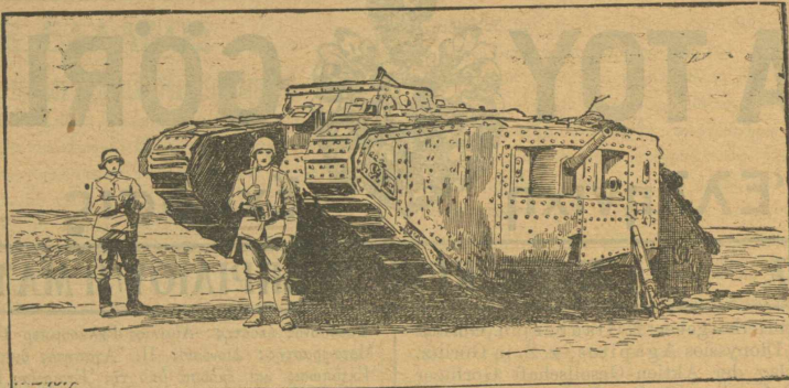
Επὶ bei Arras erbeuteter englischer Tank. 'Εν παρά τῷ Ἀρράς κυριευτὸν ἀγγλικὸν τεθωρακισμένον αὐτοκίνητον.
