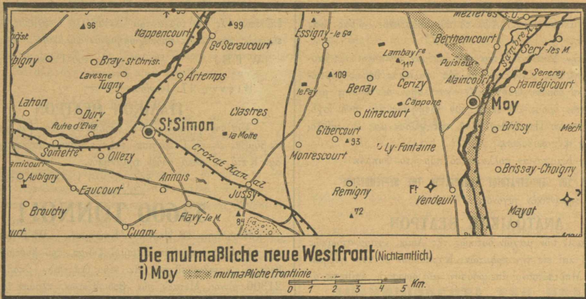
Τὸ πιθανὸν νέον δυτικὸν μέτωπον. Τμήμα Μουά. (Ἡ γραμμὴ τοῦ μετώπου δεῖκνύεται ὑπὸ τῆς ἐκ στιγμῶν συγκαμμένης κυρτοῦς.)
