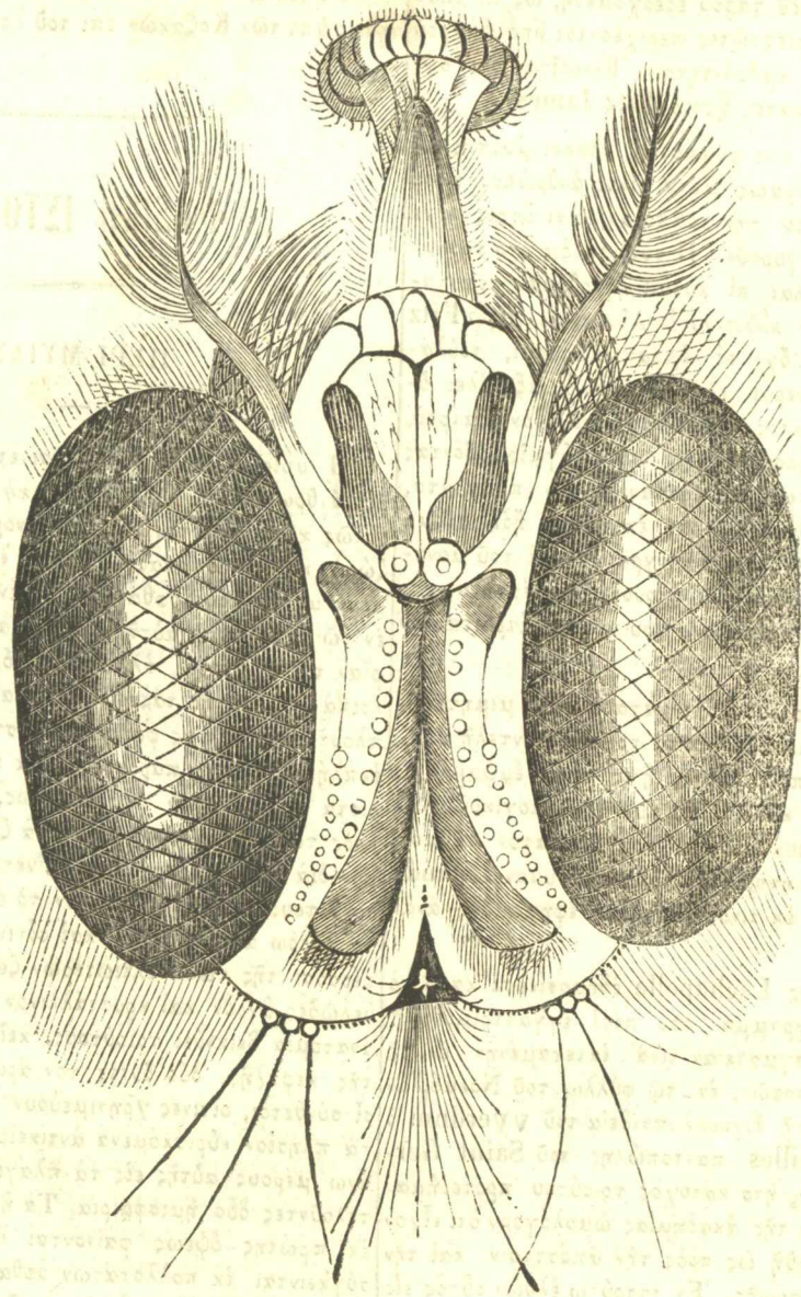
Κεφαλὴ μύιας διὰ τοῦ μικροσκοπίου.
