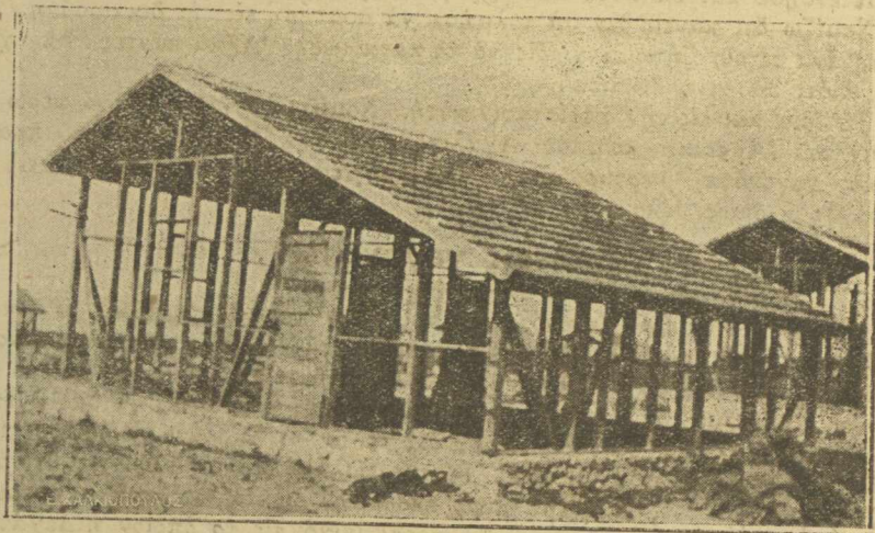
Εικών 1. Ένας ξύλινος Σκελετός σκεπασμένος, τύπου Α., όπως τον παρέδωκεν ή Δεχάτεγχε στα Λαγκαδίκια. Η Δεχάτεγχε διά τον Σκελετόν αυτόν επληρώθη λίρες 'Αγγλίας 36 και 13 σελίνια.
