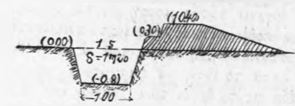
Καλυπτήριον διὰ τοῦς ὀρθίως βάλλοντας (Σχ. 2).
