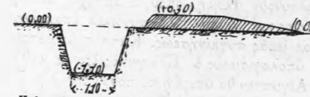
Καλυπτήριον δι' ὀρθίως βάλλοντας. Καταβασομένη κατατομή 1/100 (Σχ. 3).
