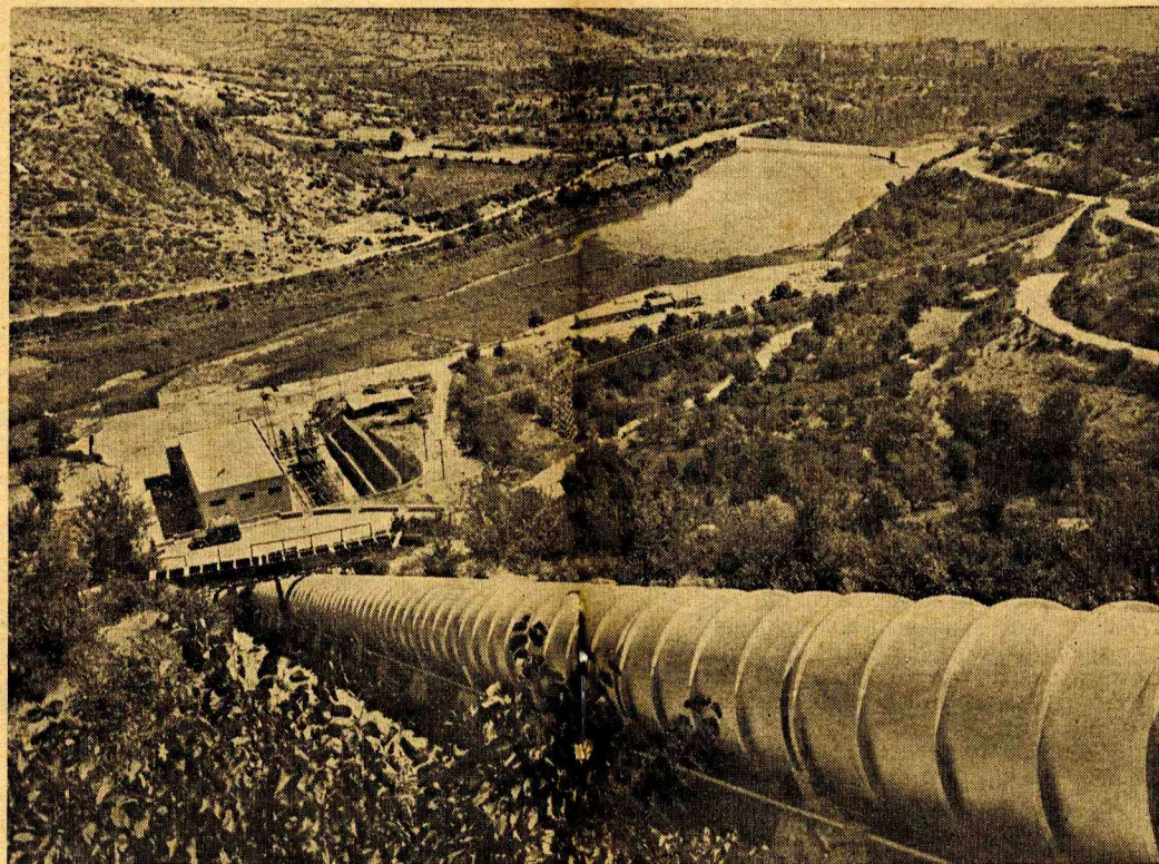
ΓΕΝΙΚΗ ΑΠΟΨΙΣ ΤΟΥ ΥΔΡΟΗΛΕΚΤΡΙΚΟΥ ΕΡΓΟΣΤΑΣΙΟΥ ΑΓΡΑ
