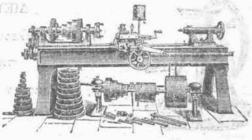
Τόρνος παντός εἶδους και μεγέθους
