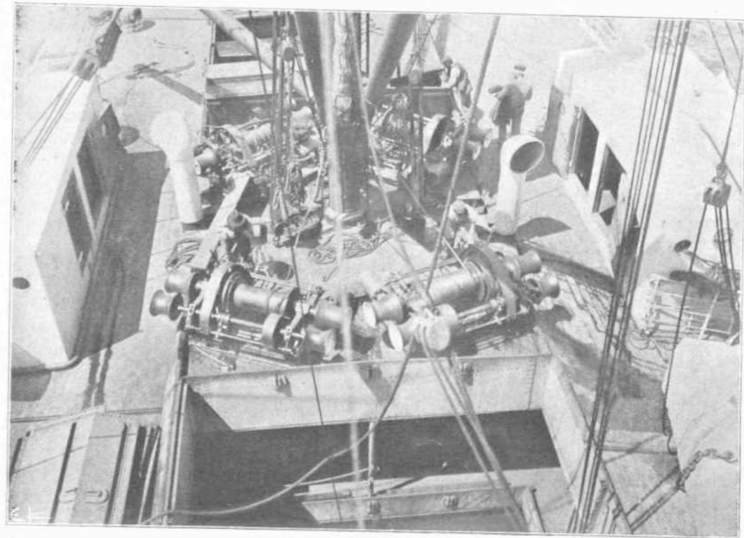
Η ΠΡΩΡΑ ΤΟΥ ΜΩΡΑΪΤΟΥ, ΜΕΤΑ ΤΟΥ ΚΥΤΟΥΣ ΚΑΘ' ΗΝ ΣΤΙΓΜΗΝ ΦΟΡΤΩΝΟΥΝ ΜΑΡΜΑΡΑ
