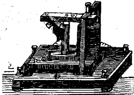
Ἡλεκτρομαγνήτης μετὰ τοῦ ὀπλισμοῦ του.
